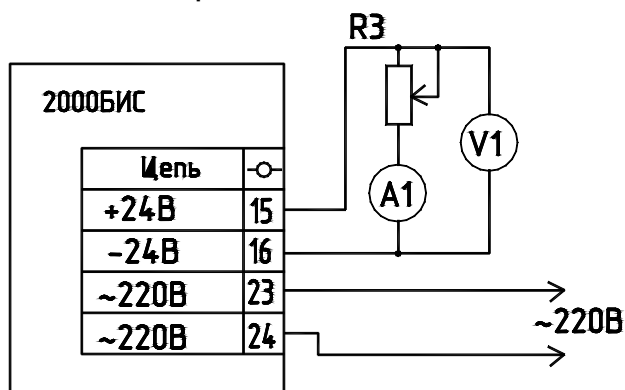
Рисунок Г.2 Схема проверки отклонения выходного напряжения ИПД
