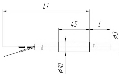
Рисунок А.4 ТНН-П-В, ТХА-П-В
