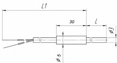
Рисунок А.3 ТПП-П-В
