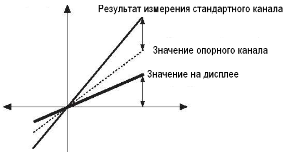
Рисунок 1 – График функции Difference
