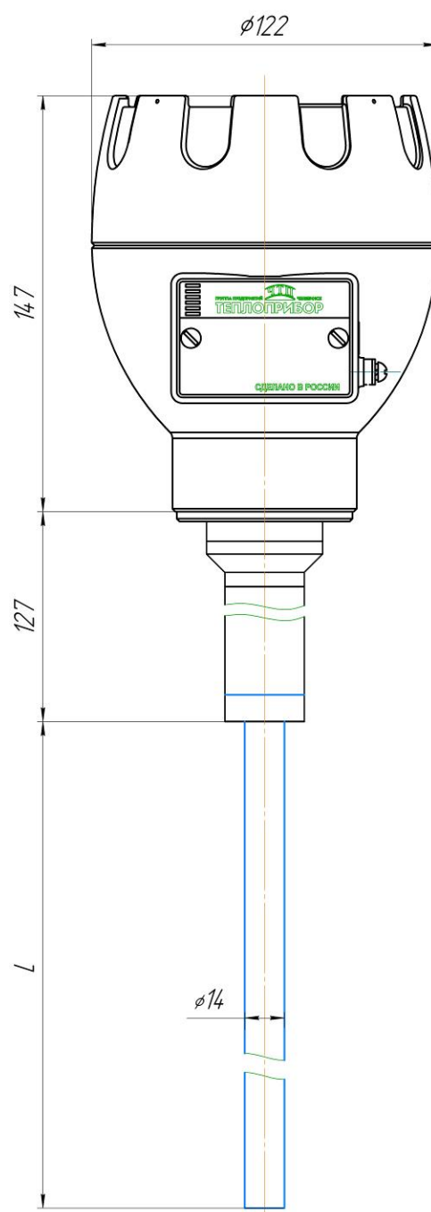
Левелтач F с стержневым зондом Ø14 мм без подключения (для байпаса)
