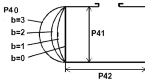
Рисунок 6 – Параметры размеров ёмкости.
